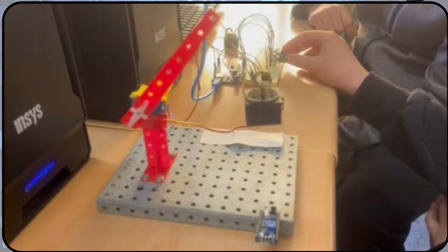
MODELO DE GRÚA CONTROLADA POR POTENCIÓMETROS.
